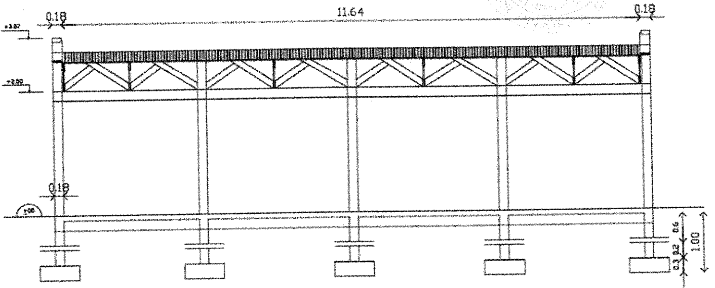
COUPE B-B
